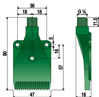
DIMENSIONI (mm) • SIZE (mm) • DIMENSIONES (mm)
